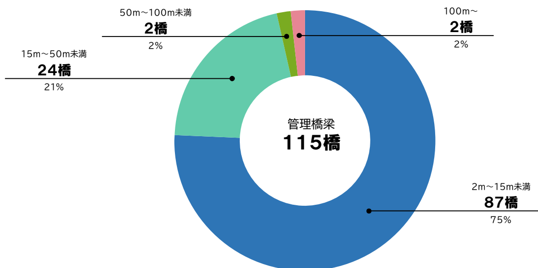
図 3 橋長別橋梁数
